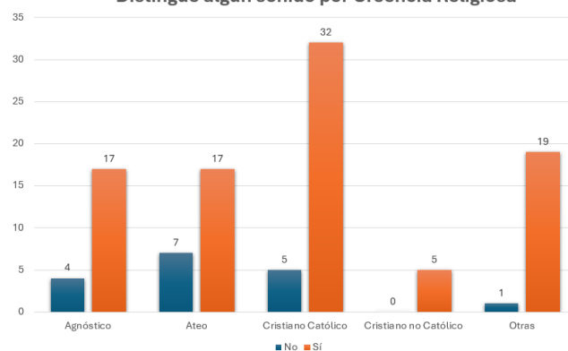
Distingue algún sonido por Creencia Religiosa
