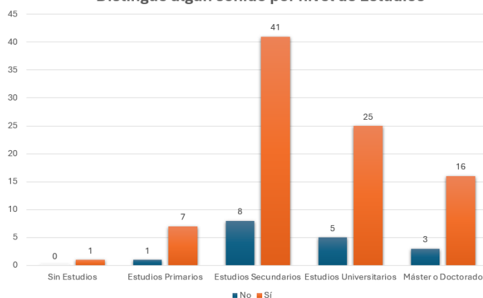
Distingue algún sonido por nivel de Estudios
