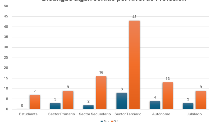
Distingue algún sonido por nivel de Profesión
