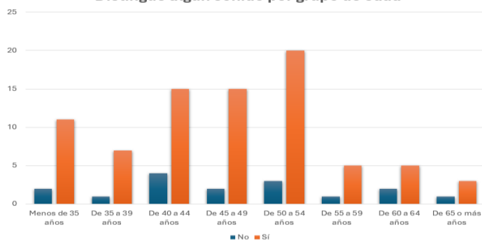
Distingue algún sonido por grupo de edad
